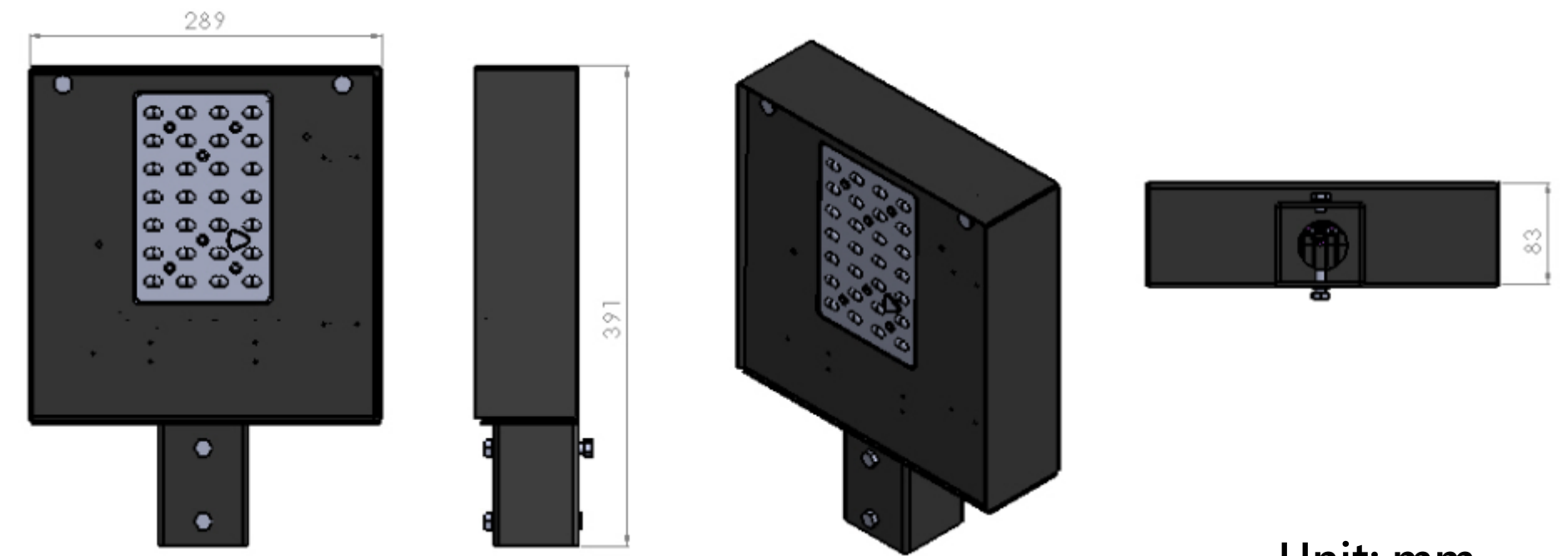
尺寸圖說：
