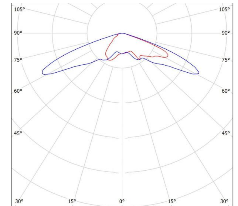
配光特性：
