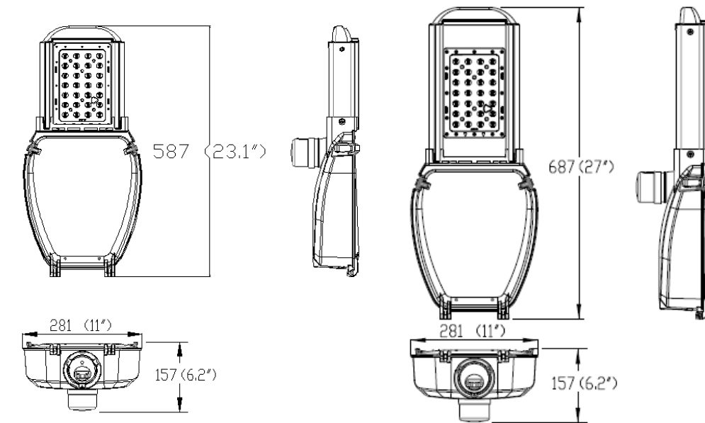
尺寸圖說：
