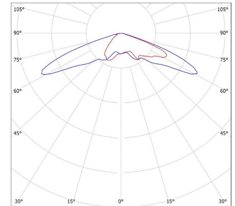
配光特性：
