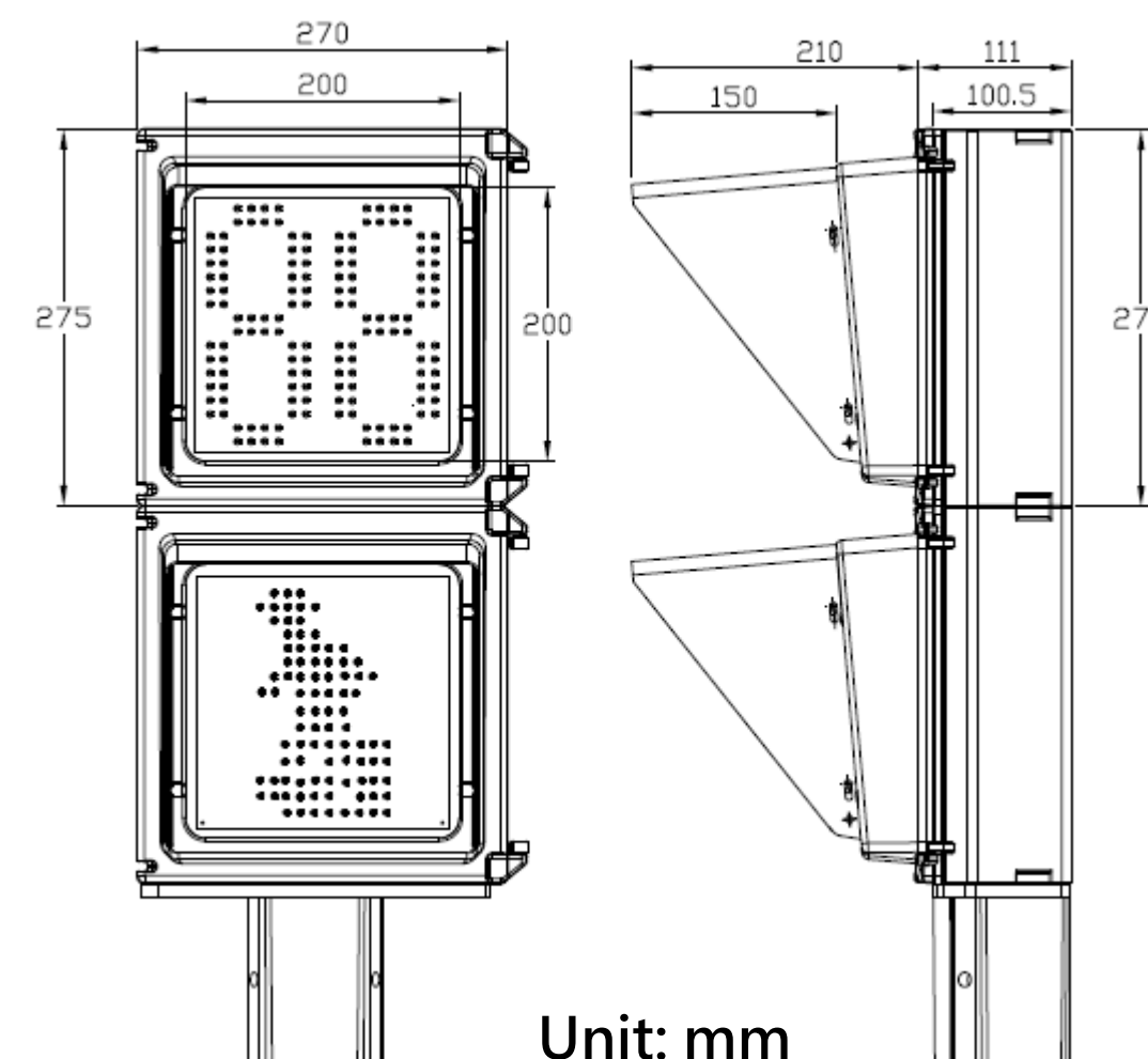
150 mm 罩簷佇立式
