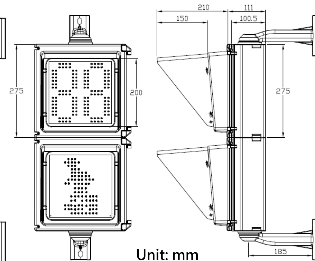
150 mm 罩簷附掛式
