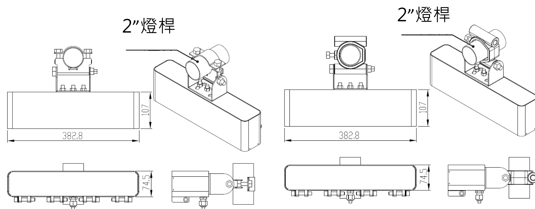
對夾式燈桿安裝
